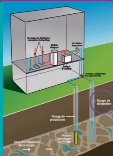
Schéma de principe d'une installation de géothermie sur nappe
